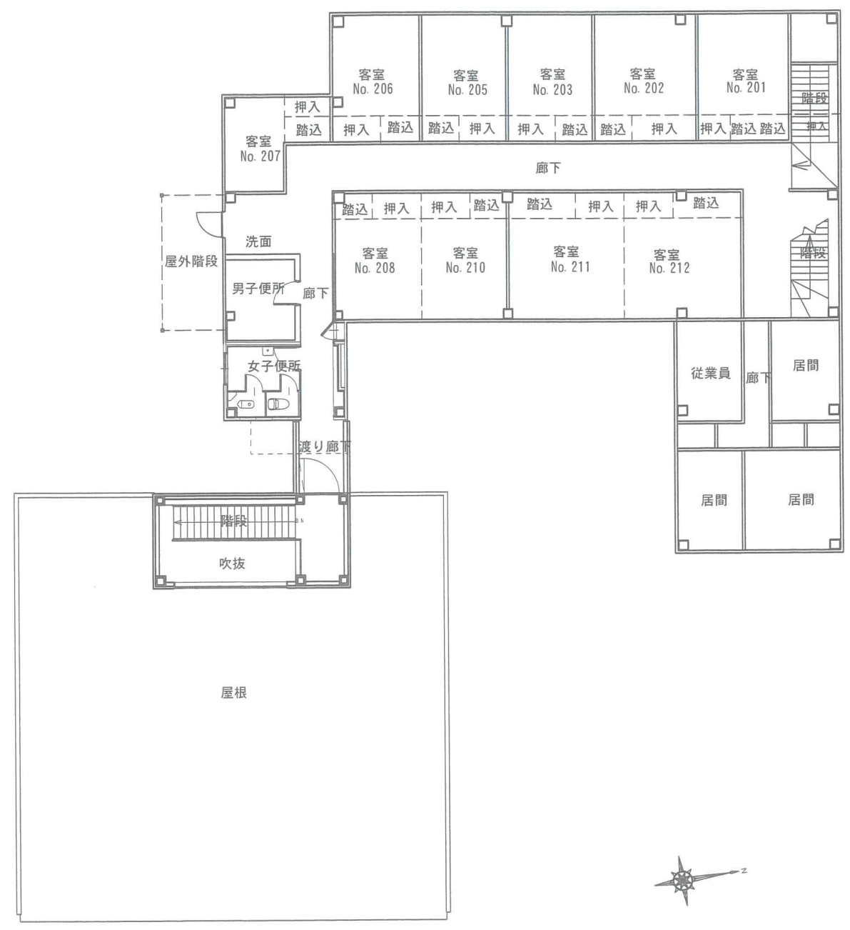
3階平面図
